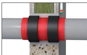
Inbouwsituatie massieve en lichte scheidingswanden \geq 100 mm
